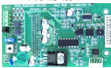
PCB-RS-485-1
