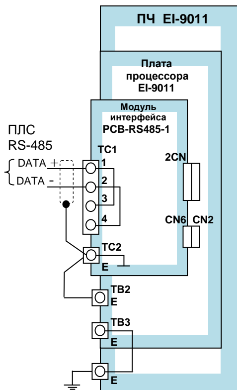
Подключение модуля PCB-RS-485-1 к ПЧ EI-9011
